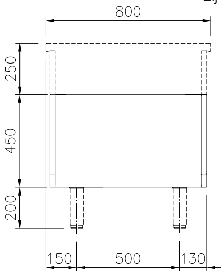
Boven aanzicht
